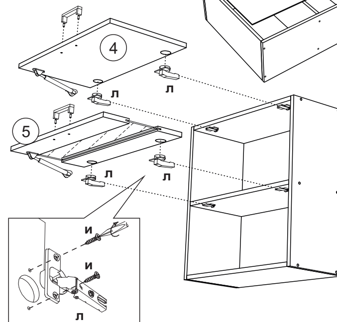
Регулировка по ширине
