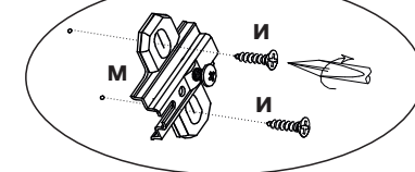
Схема крепления соединительного элемента
