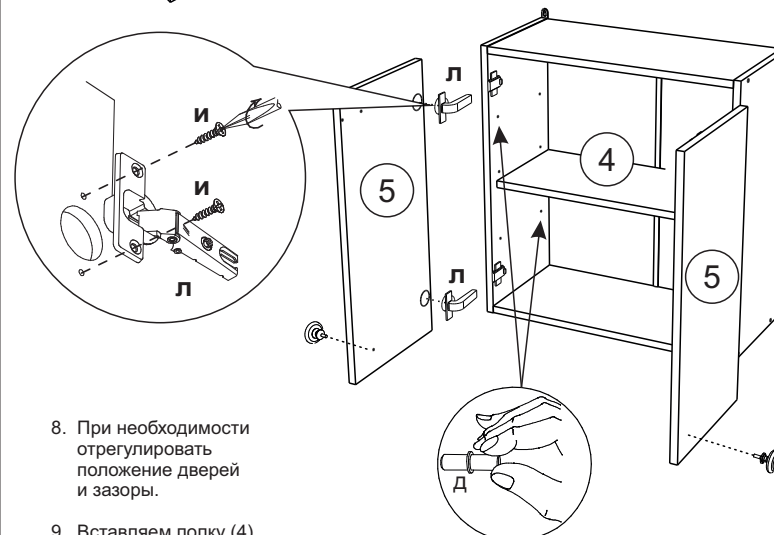
Установка полкодержателя
