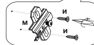
Схема крепления соед.элемента
