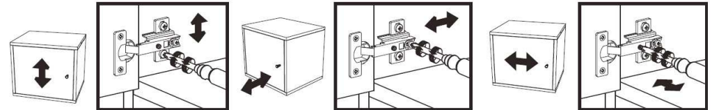
Схема регулировки фасада:
